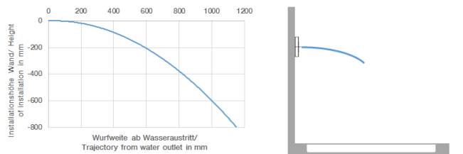
Wurfweitendiagramm
